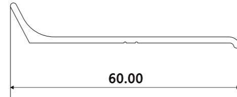
YF-3846 0.300KG/M
