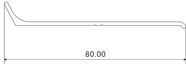
YF-4365 0.385KG/M
