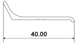
YF-3845 0.211KG/M
